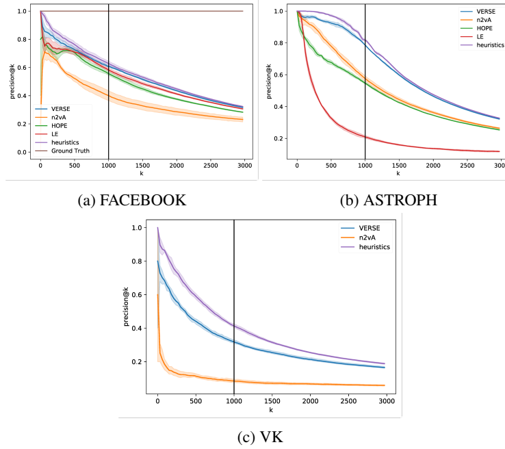
Fig. 1: Precision@k
